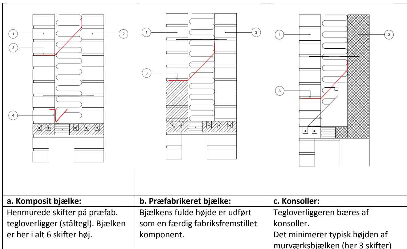
Fig. 2: Typer af bjælker i murværk og placering af fugtsikring.
