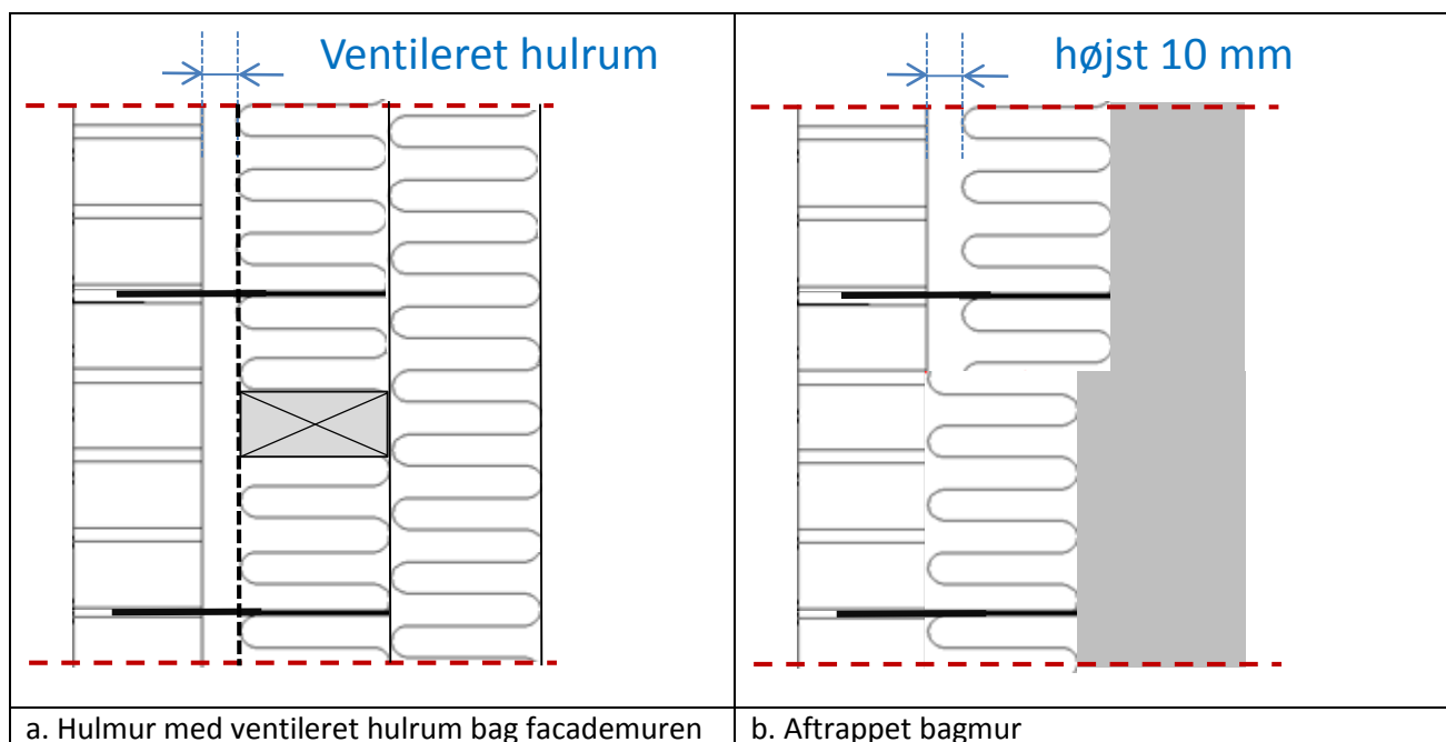
Fig. 7 Konstruktioner med ventileret hulrum på mere end 10 mm bag formuren.
